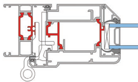
Jamb Detail
